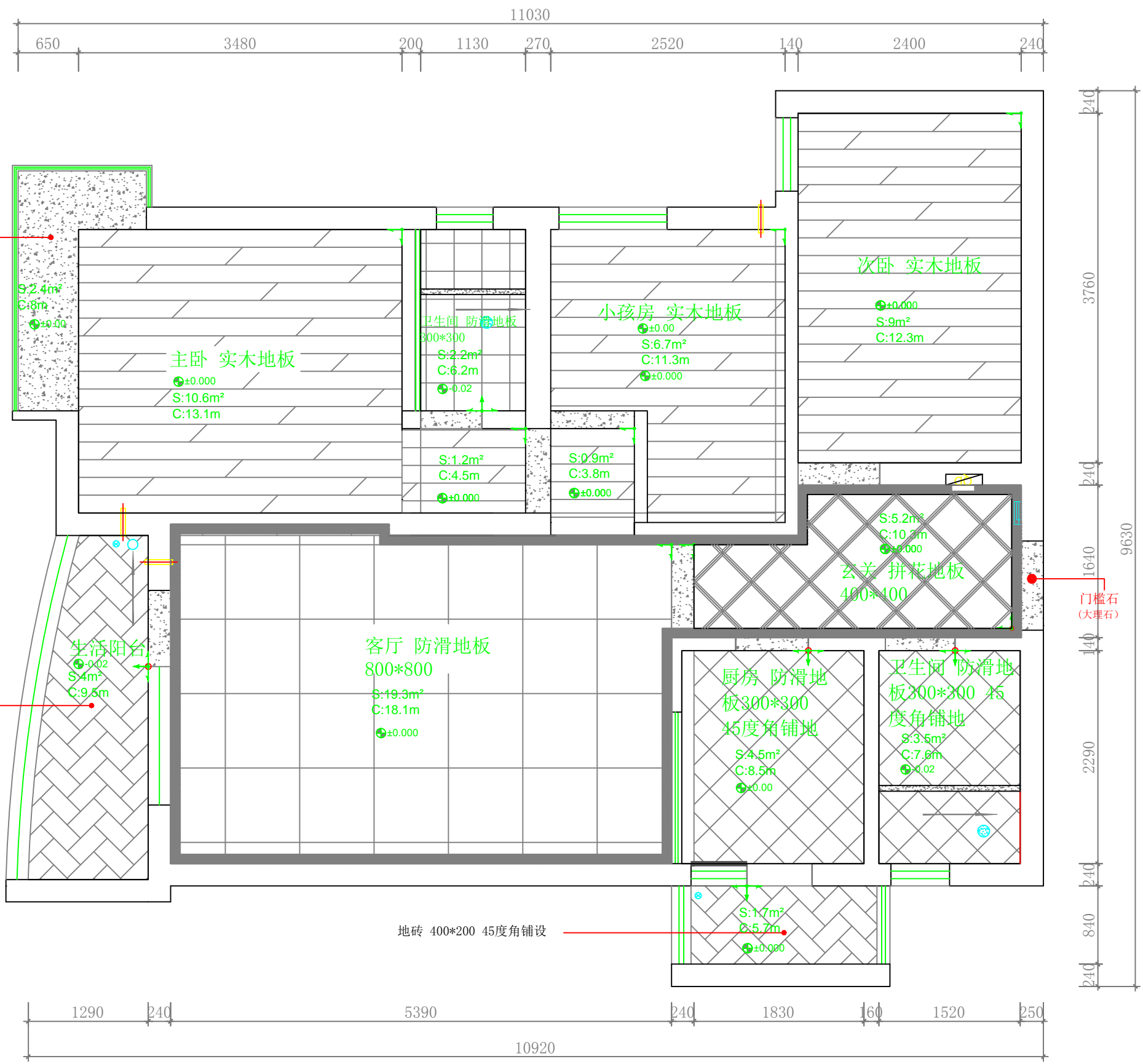
地面材质图 SCALE=1:50
